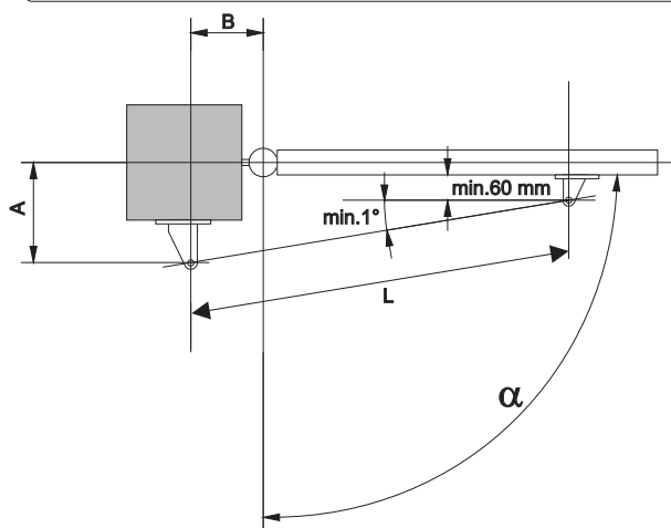
Rysunek 7. Definicje wymiarów siłowników DTM300, DTM400, DTM600 z tabelami z zalecanymi wartościami.
