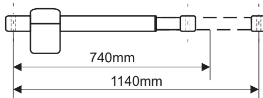
Zalecane wymiary DTM400 (mm)
