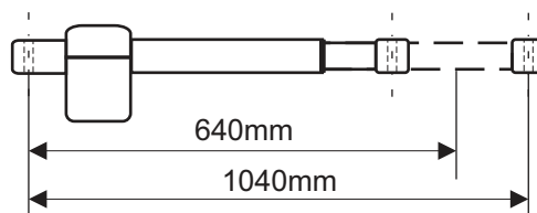
Zalecane wymiary DTM300 (mm)
