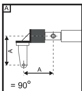
Rysunek 8. Sposoby wykonania okucia słupa
