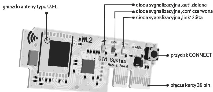
Rys. 37 Widok karty WL2.
