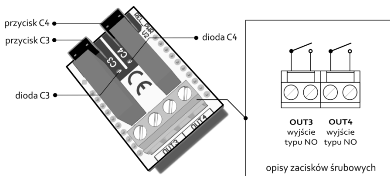
Rys. 36 Widok modułu przełącznikowego REL-2-PWR.
