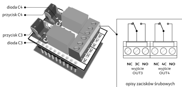
Rys. 35 Widok modułu przełącznikowego REL-2.
