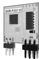
Rys. 38 Widok modułu SHR-F433
