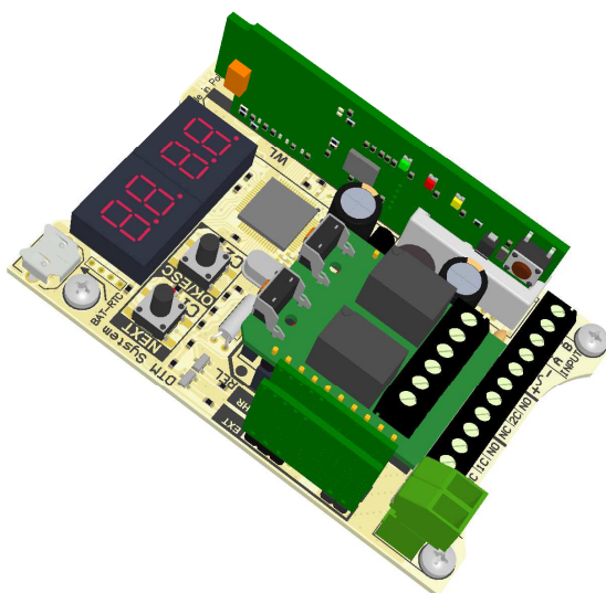
Rys. 1 Widok odbiornika FLEX868 wraz z opcjonalnymi modułami REL-2 i WL2.
