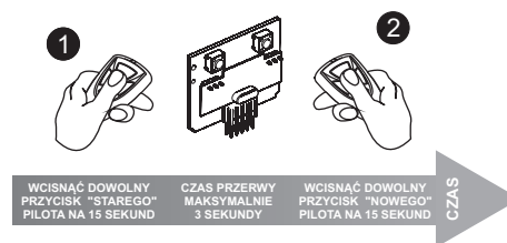
Rysunek 6. Zdalne wpisywanie pilota.
