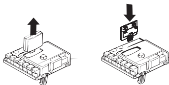
Rysunek 2. Instalacja karty radiowej S-MIX bez obudowy.
