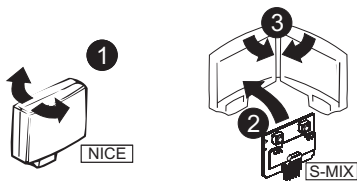
Rysunek 1. Instalacja karty radiowej S-MIX w oryginalnej obudowie radia NICE.
