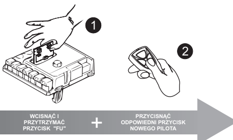
Rysunek 4. Programowanie funkcji "FU" (furtka) dla przycisku nr 2 pilota.
