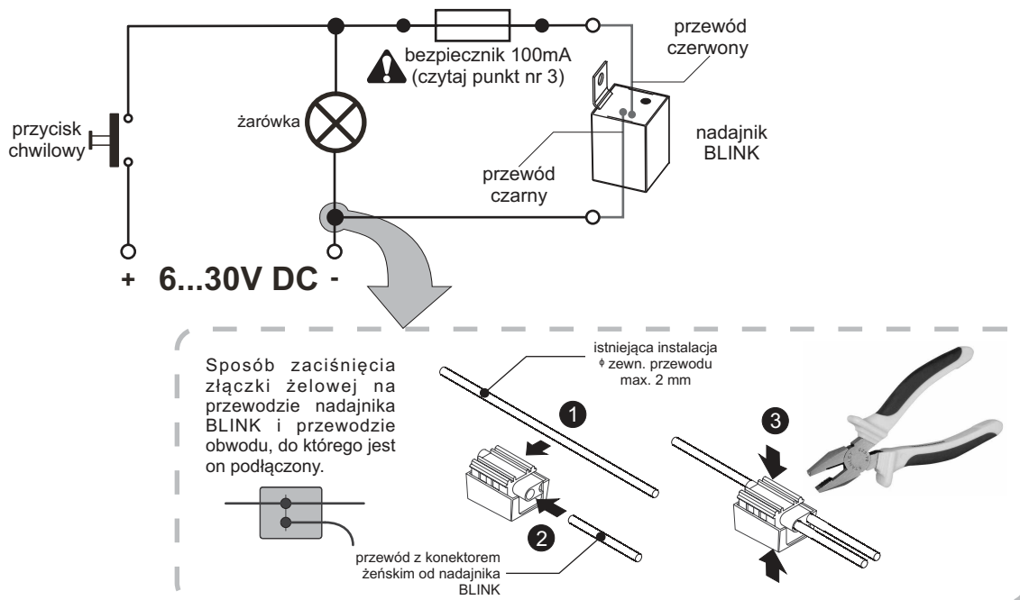
Rys. 3 Przykładowy schemat elektryczny podłączenia nadajnika BLINK, do obwodu żarówki.
