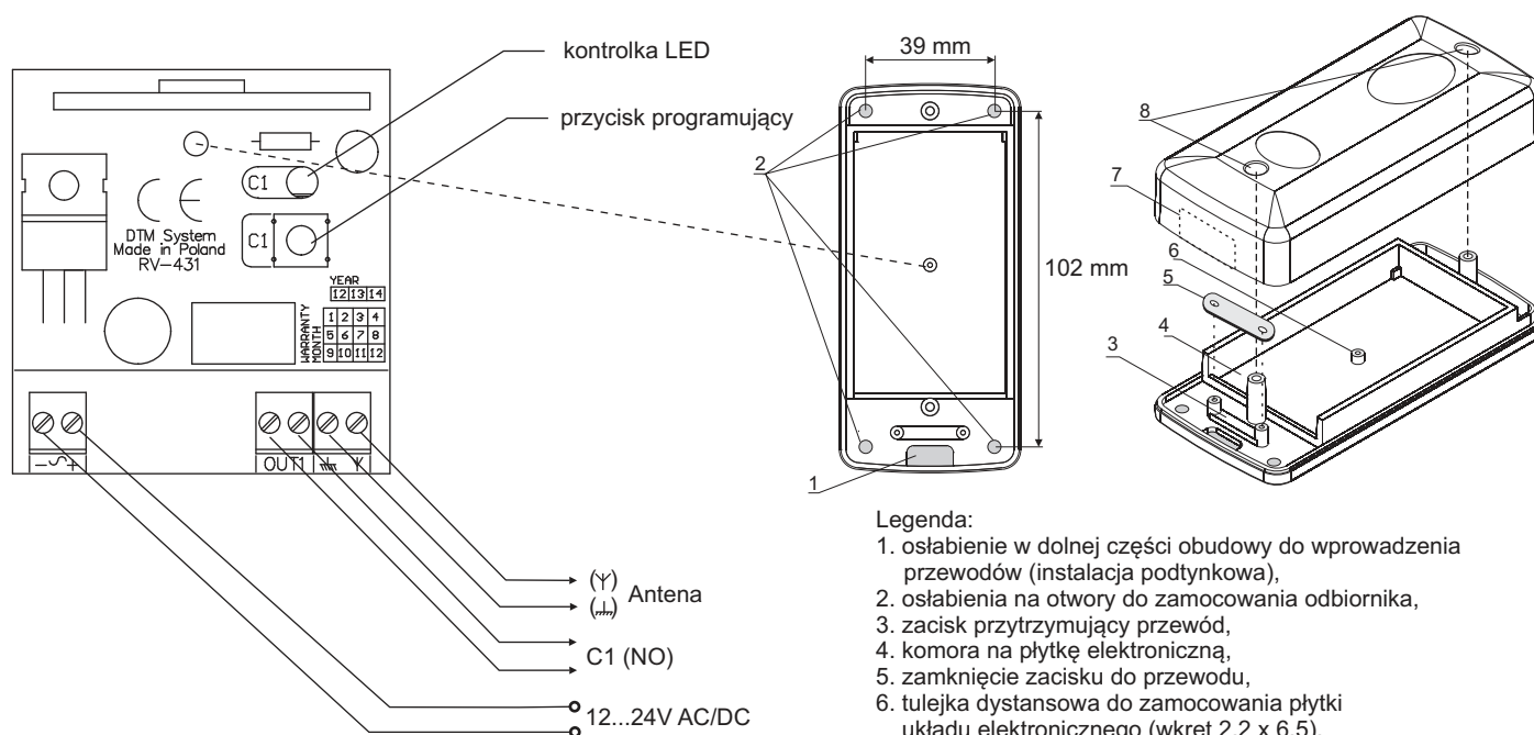
Rys. 1 Widok odbiornika radiowego wraz z obudową oraz opisem połączeń
