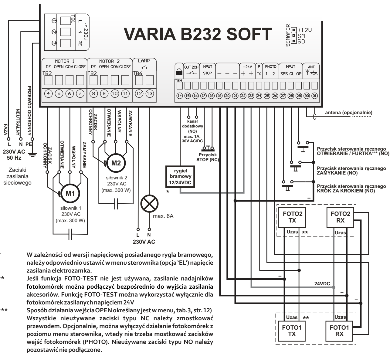
Rys.3. Sposób podłączenia zacisków sterownika VARIA B232 SOFT
