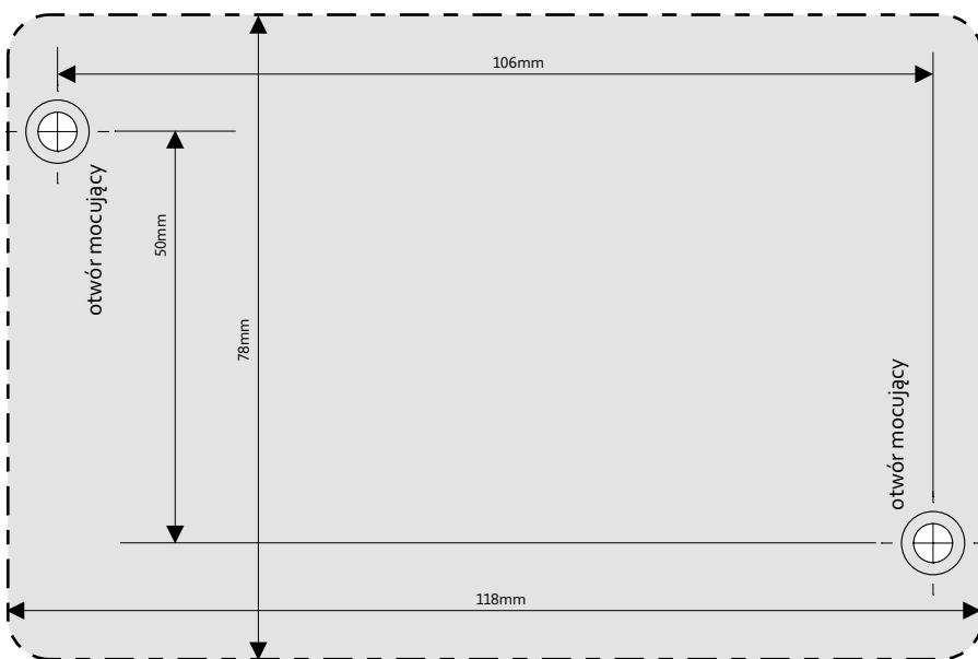
Rys.2. Rozstaw otworów mocujących w skali 1:1.
