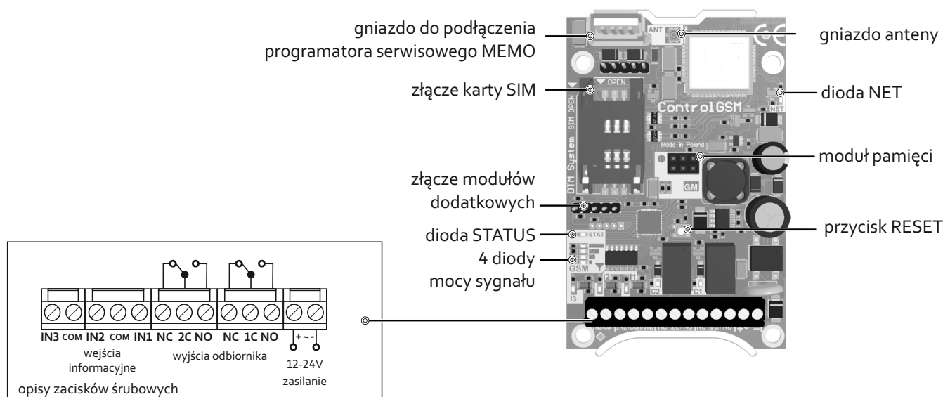
Rys.1 Widok odbiornika z opisem wyprowadzeń.
