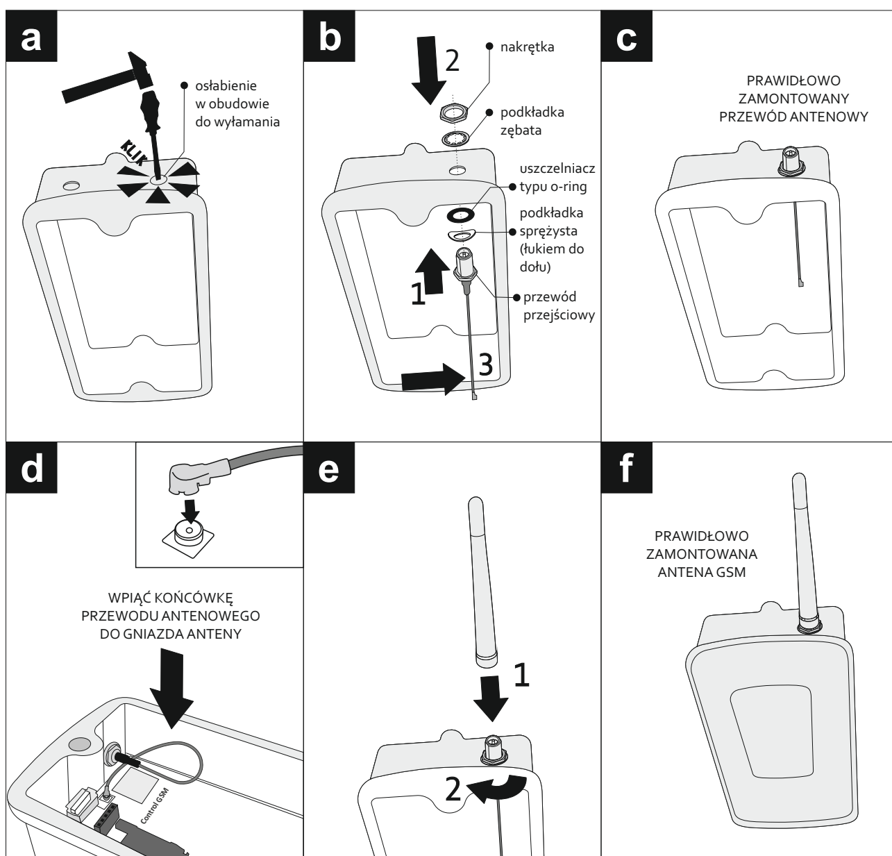
Rys.2 Montaż anteny GSM w odbiorniku.
