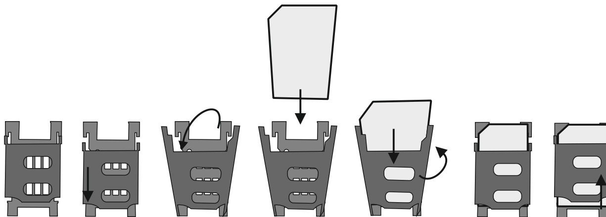
Rys.3 Instalacja karty Mini SIM w złączu odbiornika.
