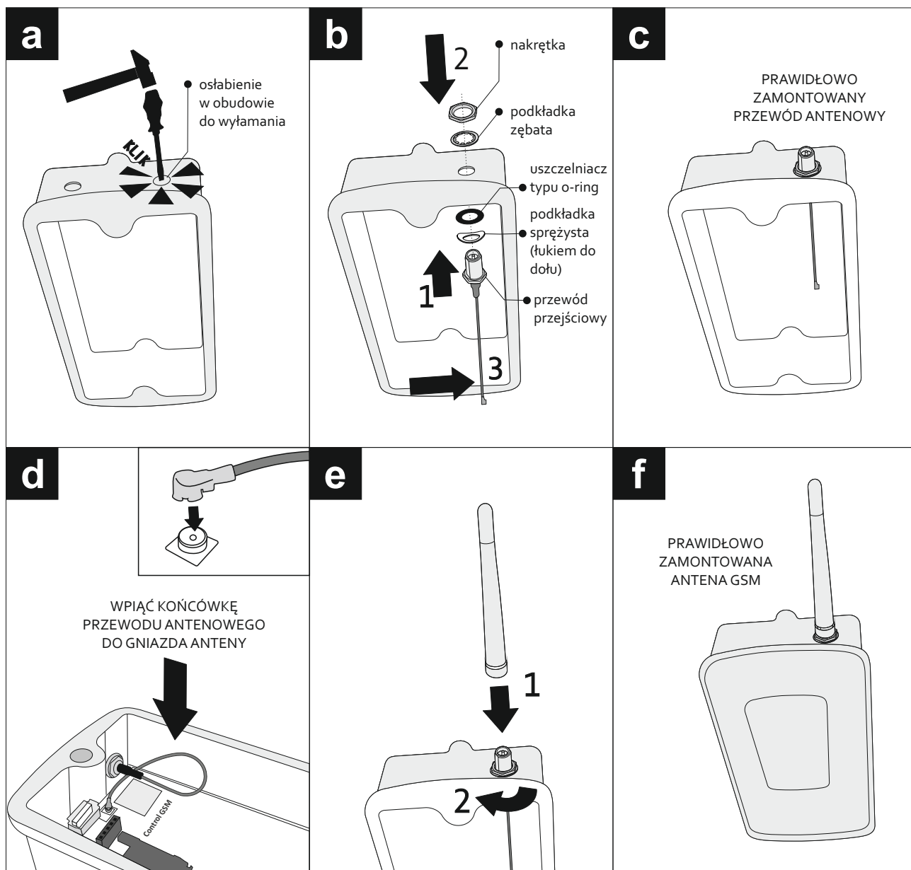
Rys.2 Montaż anteny GSM w odbiorniku.
