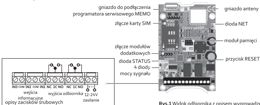
Rys.1 Widok odbiornika z opisem wyprowadzeń.
