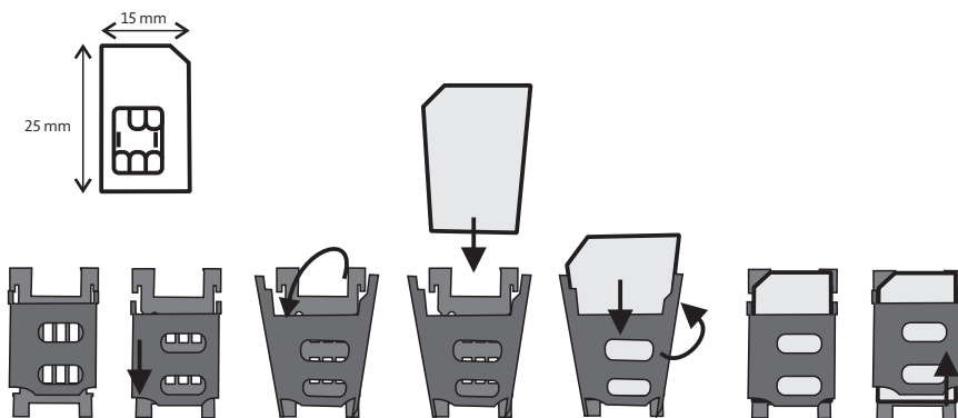
Rys.3 Instalacja karty Mini SIM w złączu odbiornika.
