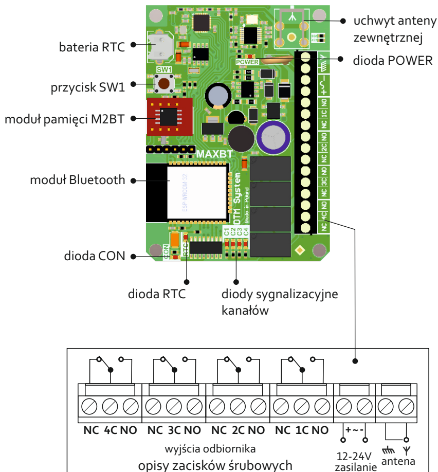
Rys. 2. Widok płyty głównej odbiornika z opisem wyprowadzeń i głównych elementów funkcjonalnych.
